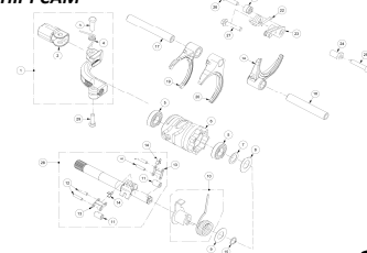
SELECTOR DE CAMBIO SHIFT CAM
