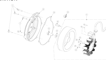
ENCENDIDO IGNITION
