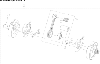
CIGUEÑAL CRANKSHAFT
